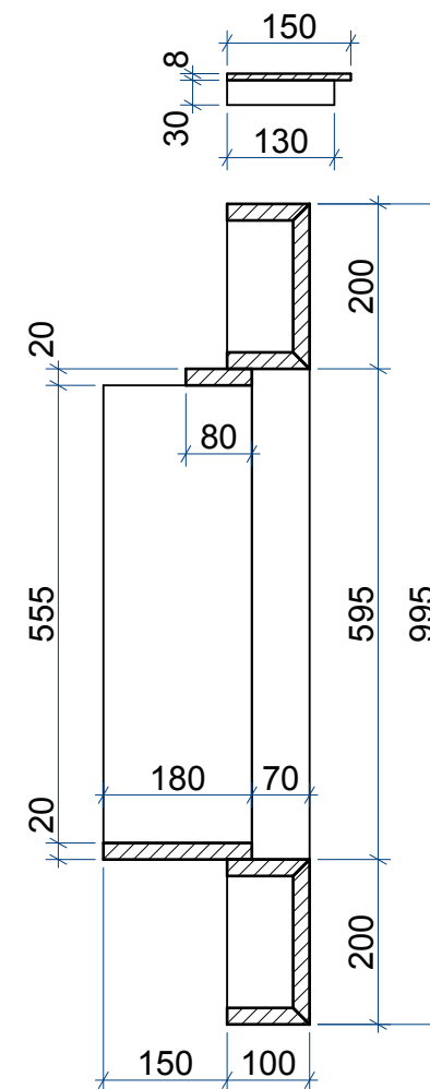
Сечение 2-2
